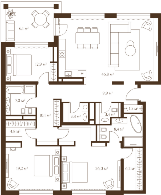
Дом №7 | Секция 5 | 4 этаж | 166,1 м²
