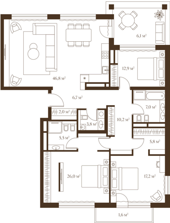
Дом №7 | Секция 1 | 7 этаж | 151,6 м²
