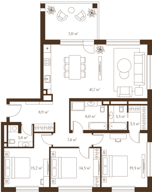
Дом №8, 9, 10 | 3 этаж | 133,0 м²
