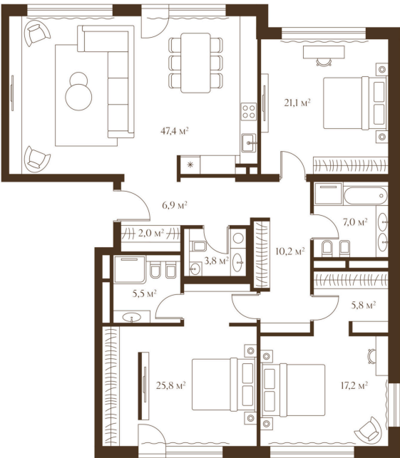
Дом №7 | Секция 2, 6 | 1 этаж | 152,7 м²
